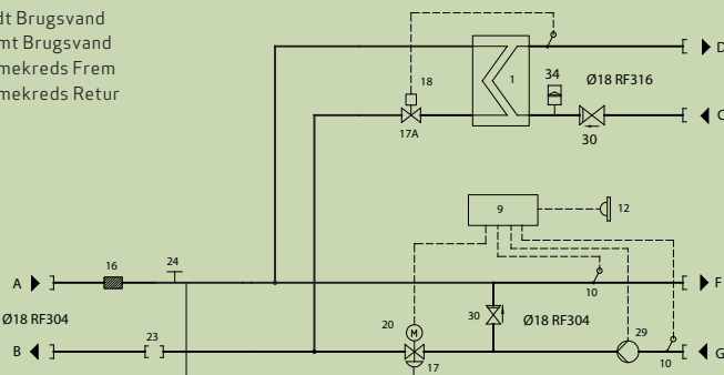
METRO SYSTEM 4 SLIMLINE MINI TERMISK
