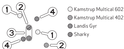
4. Energimåler (medfølger ikke) monteres i de markerede huller (se nedenfor).
