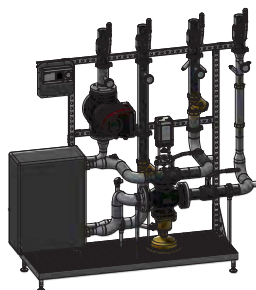
METRO VXT TYPE 5 300 - 450 kW METRO-nr.: 0129201830 VVS-nr.: 375284005
