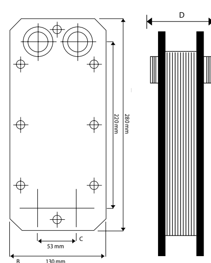
Målskitse R7xx
