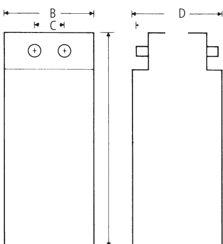
Målskitse 2720/2xx-xx
