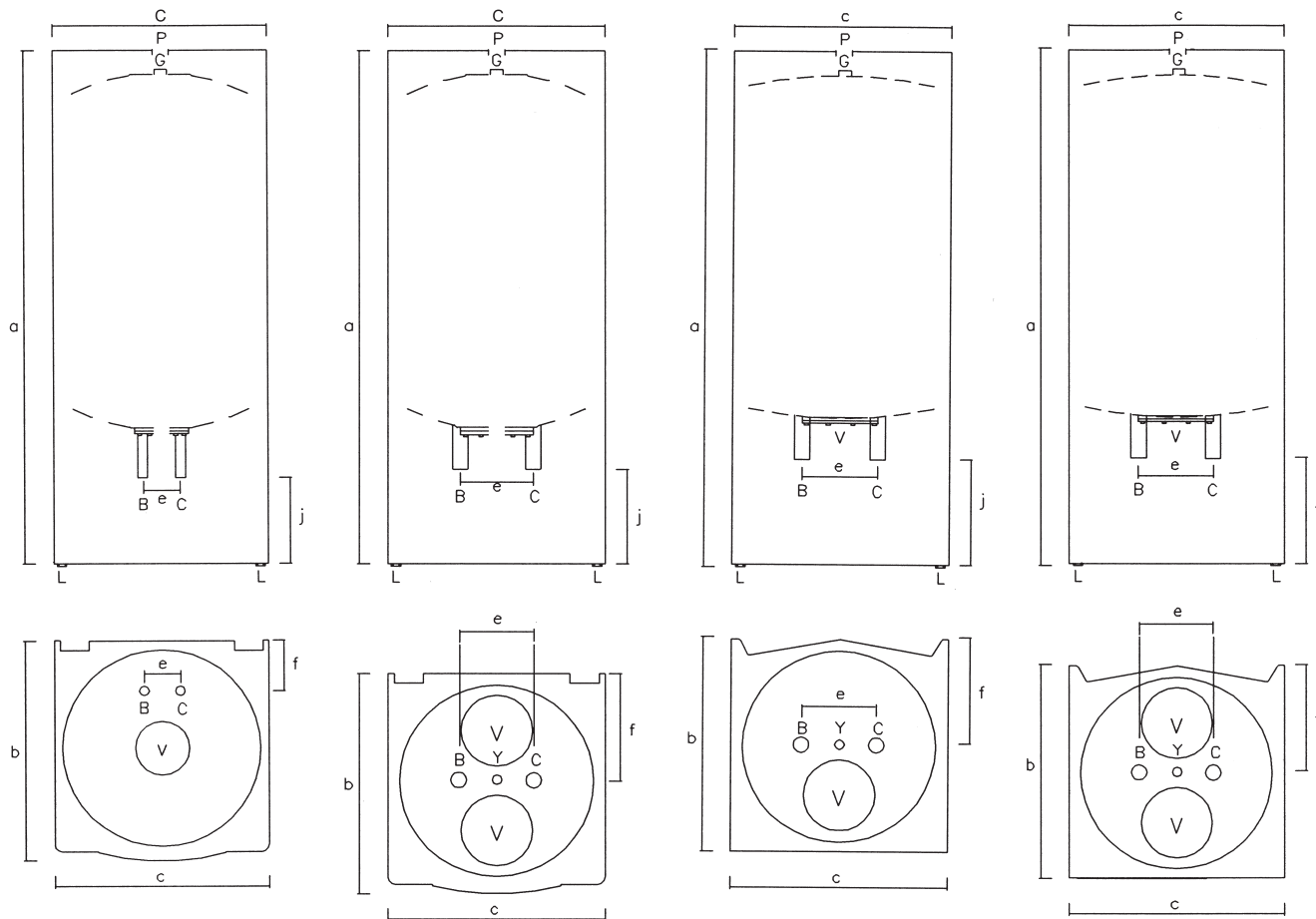
Vandvarmere 15 kW
